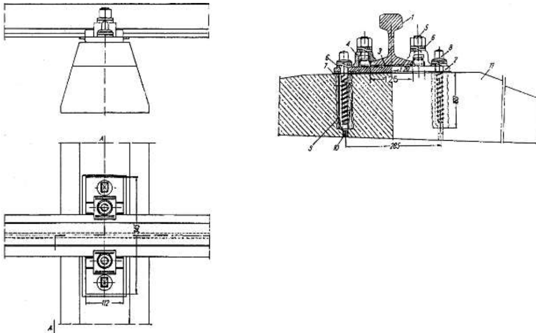
Rys.1 Przytwierdzenie typu K szyny S49(49E1) do podkładów betonowych
