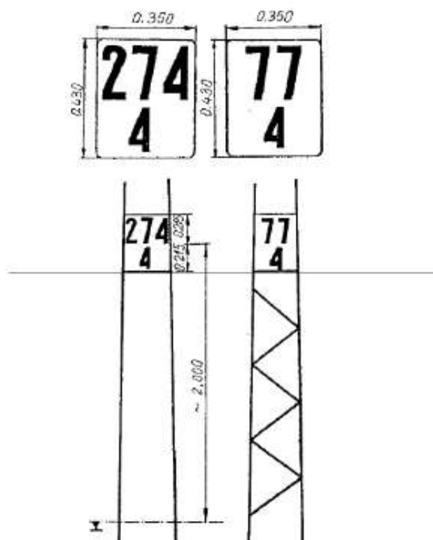
Rys.1 Znaki kilometrowe i hektometrowe na liniach zelektryfikowanych
