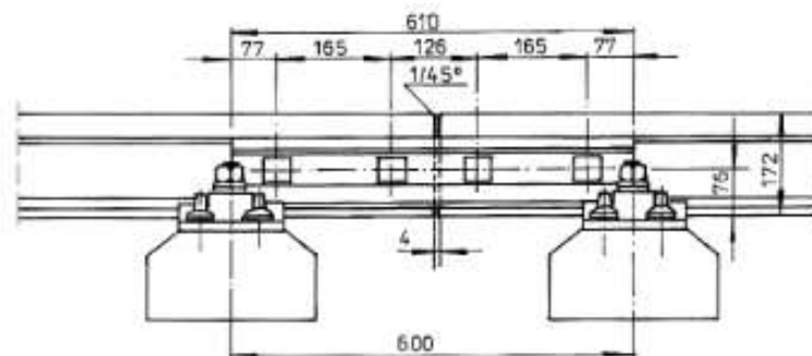
Rys. 9 Złącze szynowe izolowane klejono-sprężone z łubkami czterootworowymi
