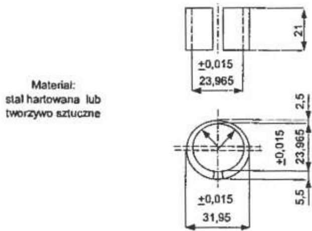
Rys. 7. Tulejki mimośrodowe.
