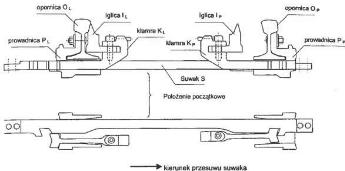
Rys. 12. Zamknięcie nastawcze suwakowe – budowa.
