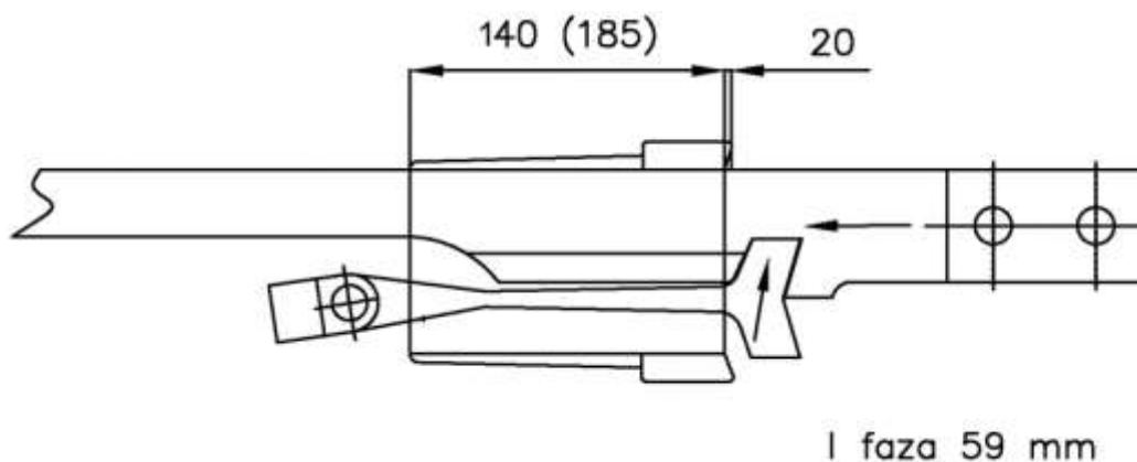
Rys. 18. Suwakowe zamknięcie nastawcze – końcowa faza przesuwu suwaka.
