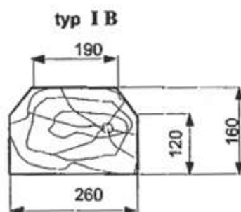
Rys. 5. Przekrój poprzeczny podrozjazdnic drewnianych stosowanych na bocznicach (typu belkowego)
