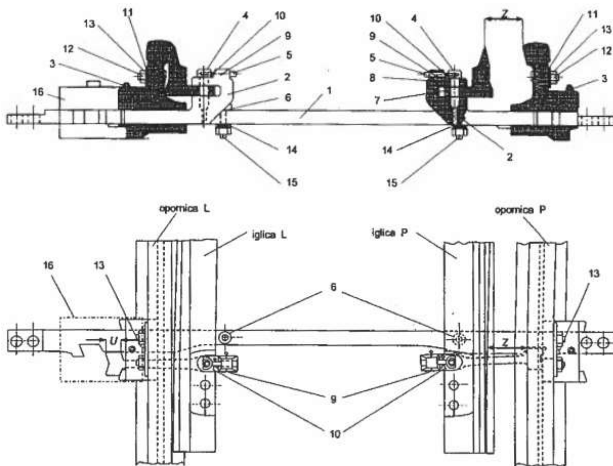
Rys. 7. Tulejki mimośrodowe.
