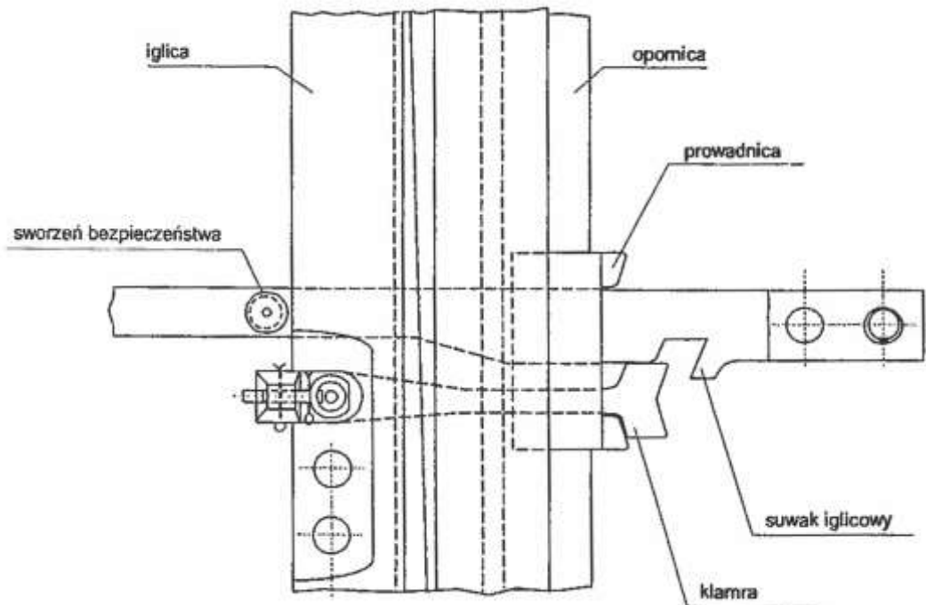
Rys. 11. Suwak iglicowy ze sworzniem bezpieczeństwa.
