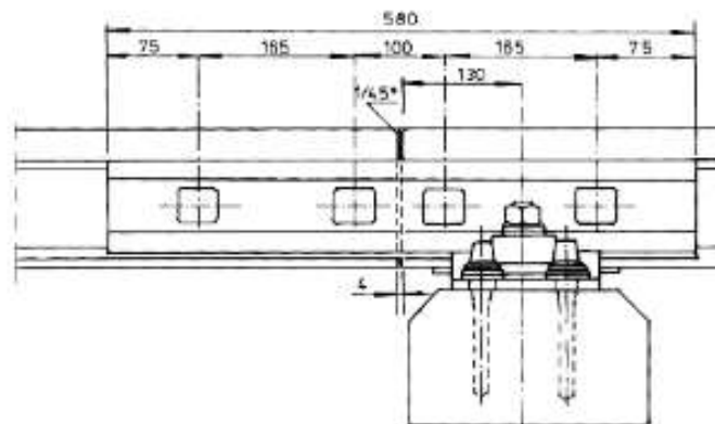
Rys.10 Złącze szynowe izolowane klejono-sprężone z łubkami czterootworowymi
