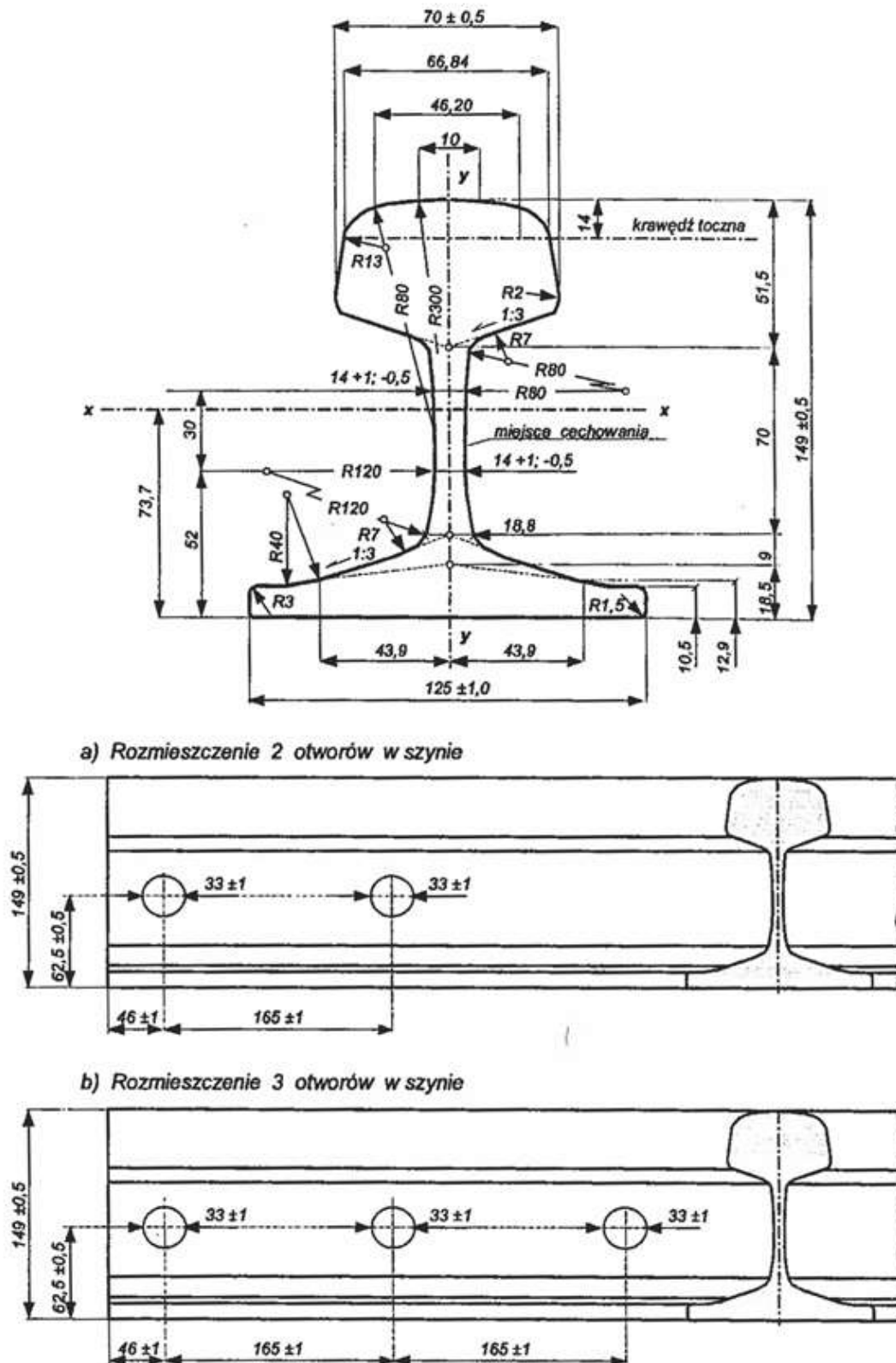
Rys. 1. Przekrój poprzeczny szyny S49
